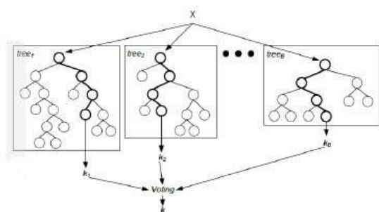
Gambar 1 Arsitektur umum Random Forest (Verikas et al. 2011).
